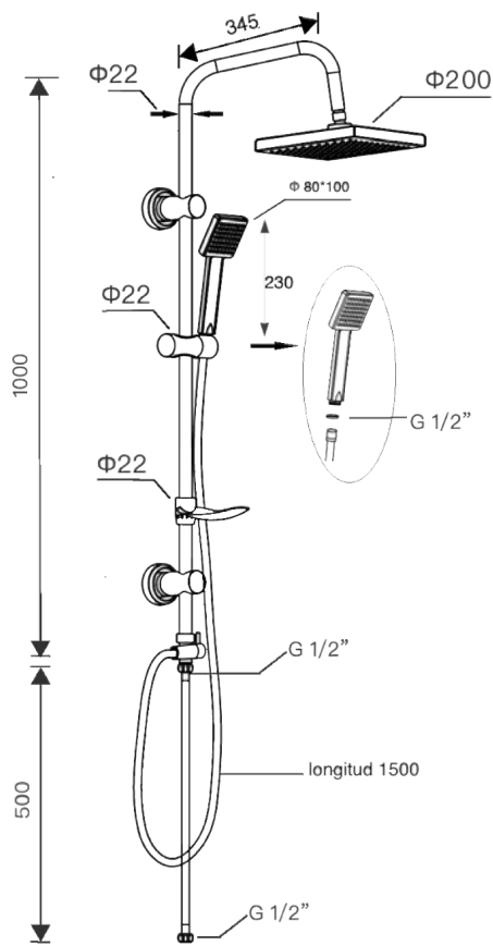
PLANO TÉCNICO
