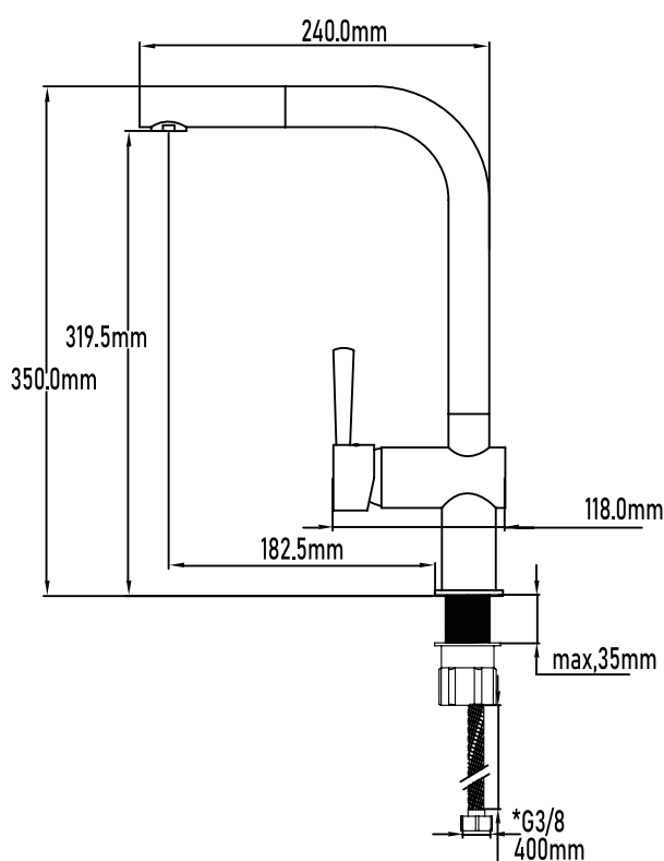
PLANO TÉCNICO
