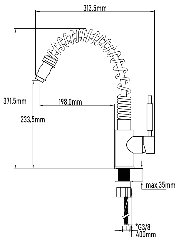
PLANO TÉCNICO
