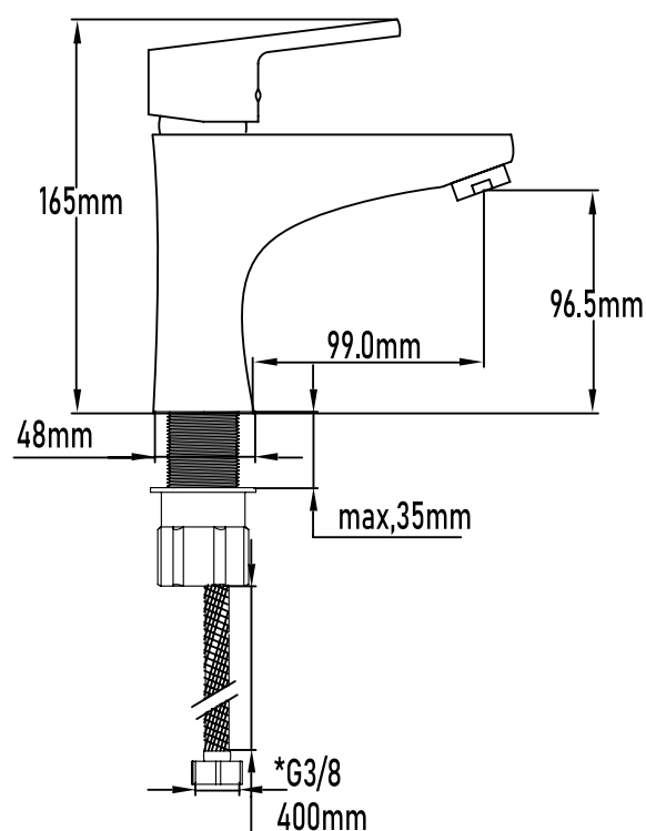
PLANO TÉCNICO
