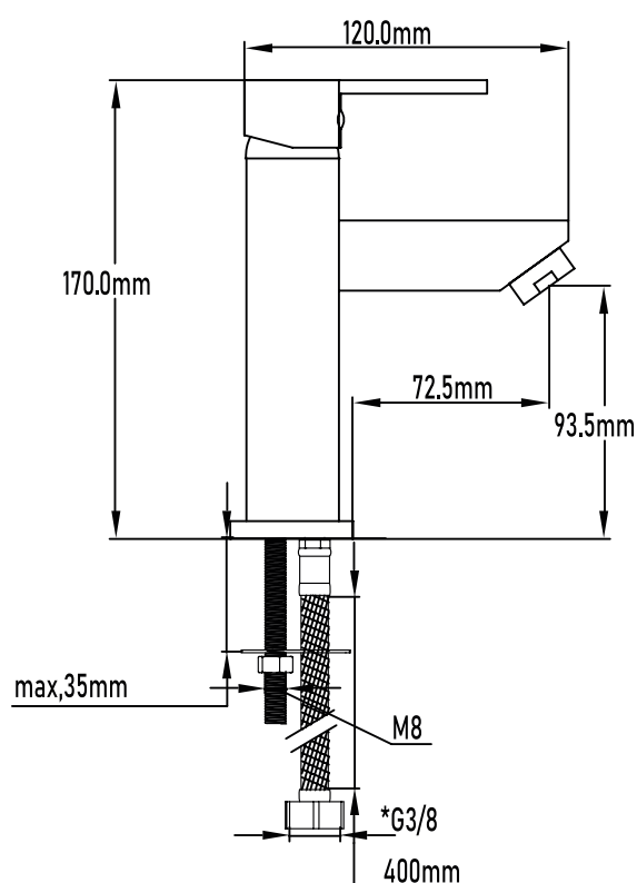
PLANO TÉCNICO
